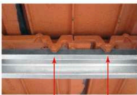
Pengait pada reng kuat dan kokoh
